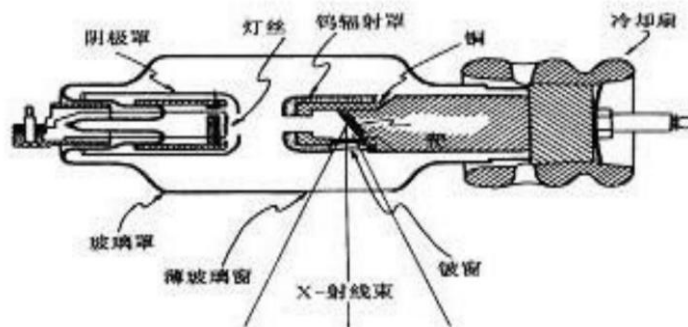
图 9-4 X 射线管基本结构示意图
