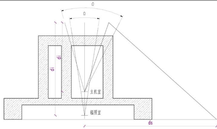
图 11-6 屋顶立角示意图
