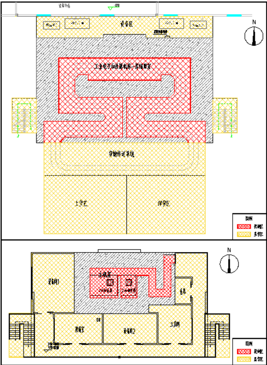
图 10-1 工业电子加速器使用场所两区划分示意图
