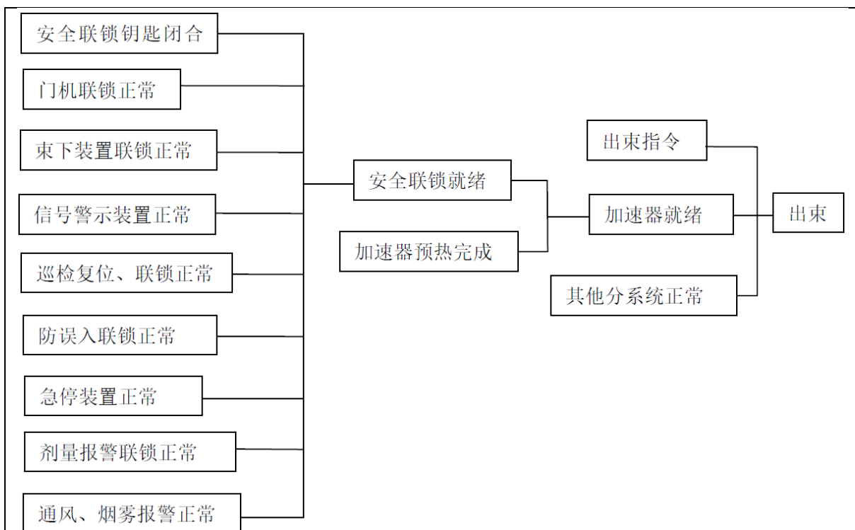
图 10-6 安全联锁设施逻辑示意图
