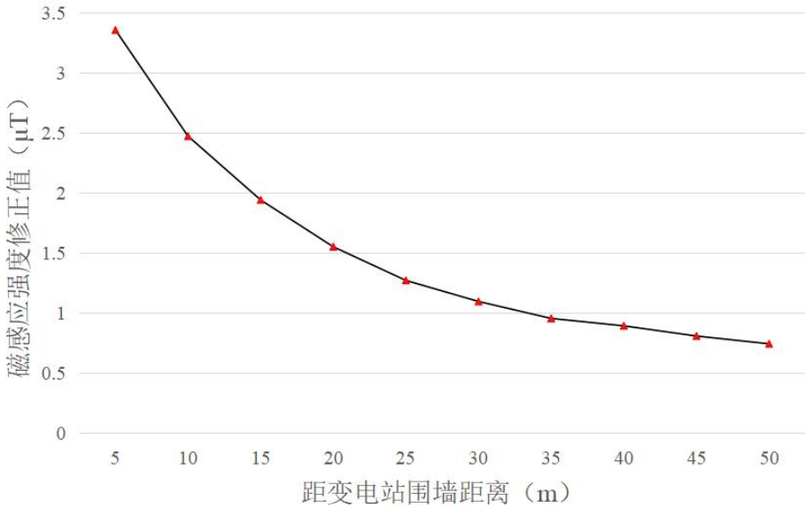
图 6-2 广都 500kV 变电站南侧衰减断面监测离地面 1.5m 高度磁感应强度分布图 从表 6-7 和图 6-1 可见,广都 500kV 变电站衰减断面监测值最大工频电场强度为
